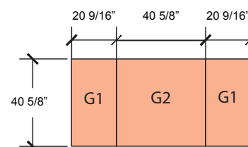
Elevation G1 & G2 (Sintra)
