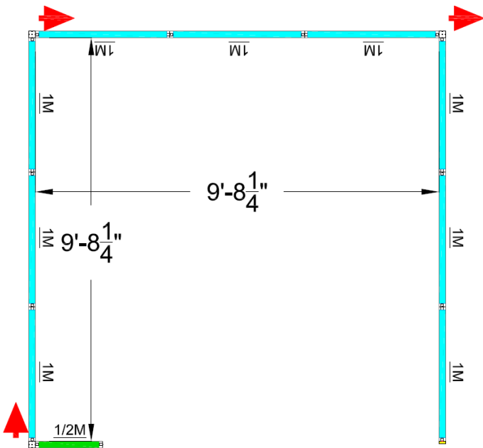
10x10 Actual Working Space Layout
