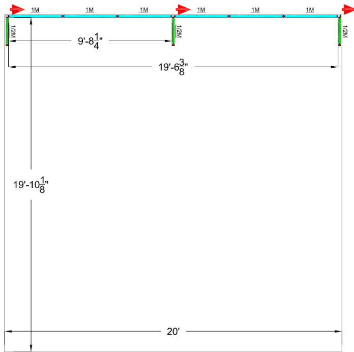
20x20 Actual Working Space Layout
